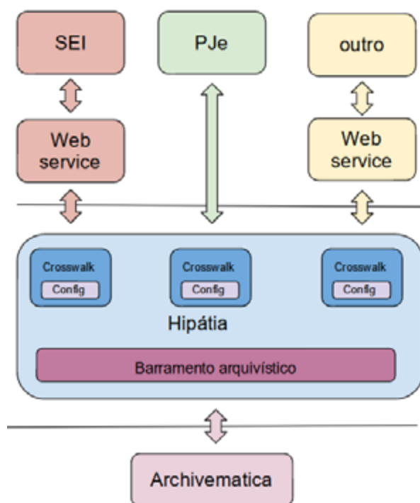
Figura 2 – Estrutura do Hipátia
